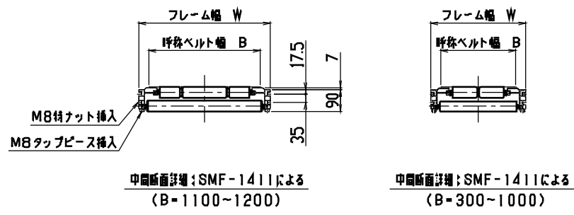
幅関係寸法
