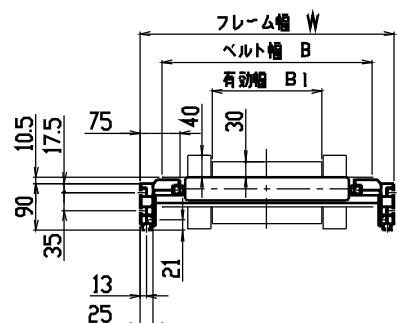
中間断面図
