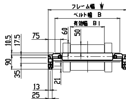
中間断面図
