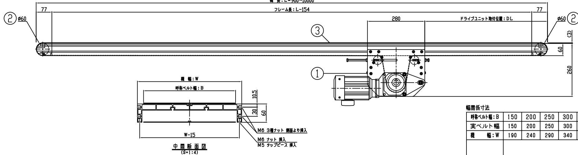
ドライブユニット取付位置
