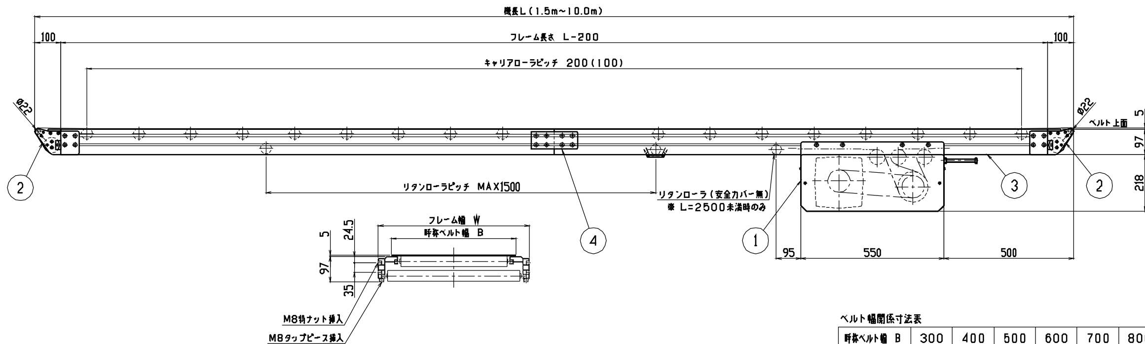
中間断面詳細：SMF-1411による
