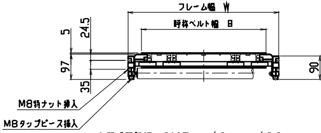
中間断面詳細; SMF-1421, 1422による
