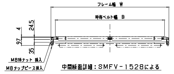
幅関係寸法
