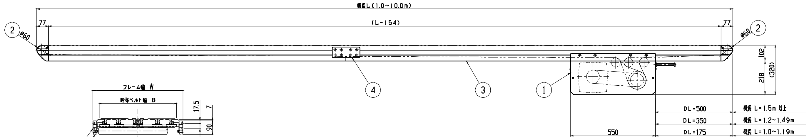
幅関係寸法
