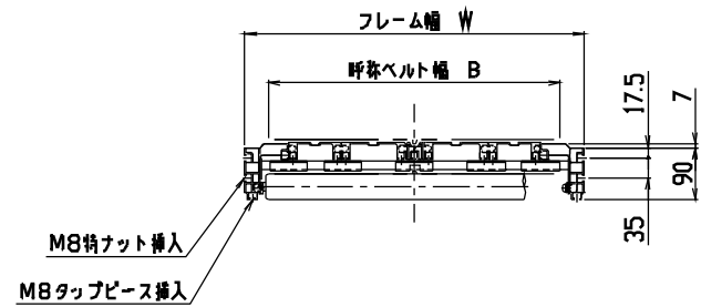
中間断面詳細: SMFV-1521, 1522による (B=300~1200)
