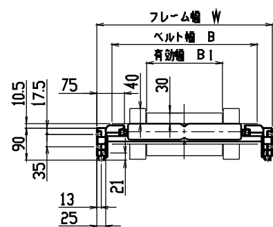
中間断面図
