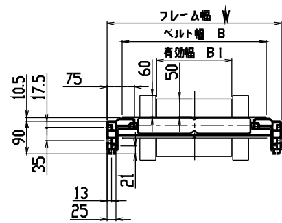
中間断面図
