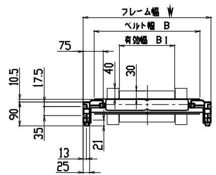
中間断面図
